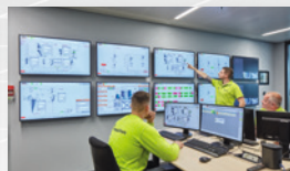
MES systems
